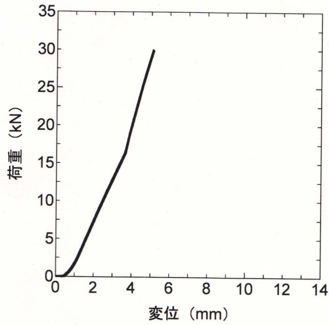
図 4 圧縮試験結果
