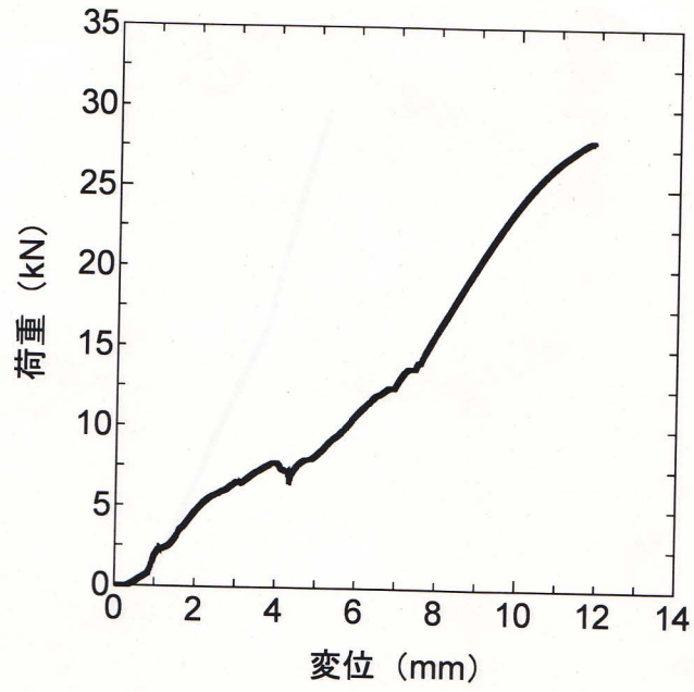
図 2 引張試験結果
