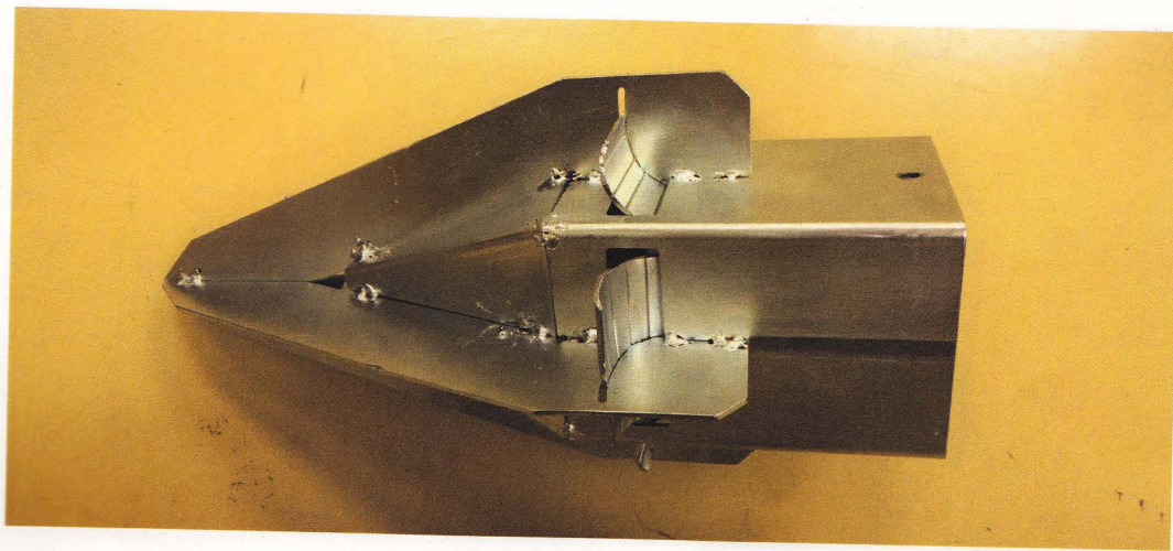
図 3 引張試験後の状態
